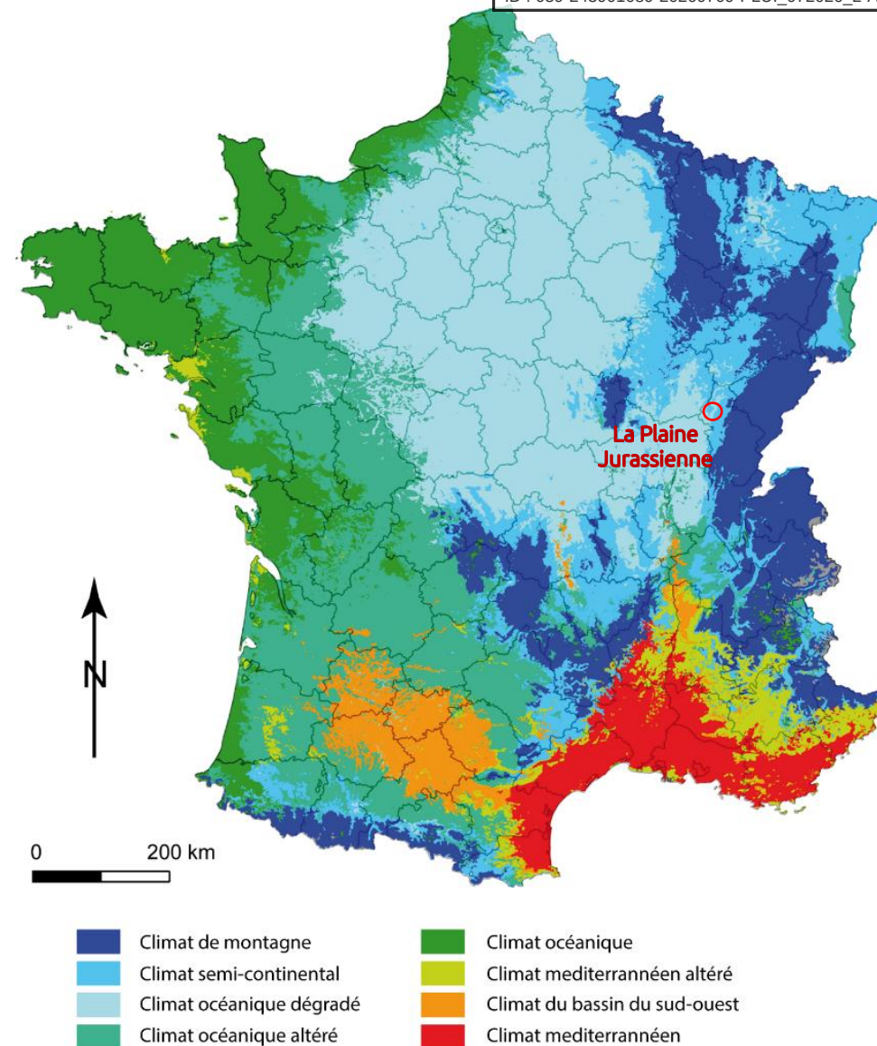
Carte 5 : Climats en France - Source Cybergeo
