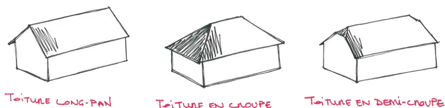
Figure 157 : Schéma des formes de toiture - Source CAUE 39
