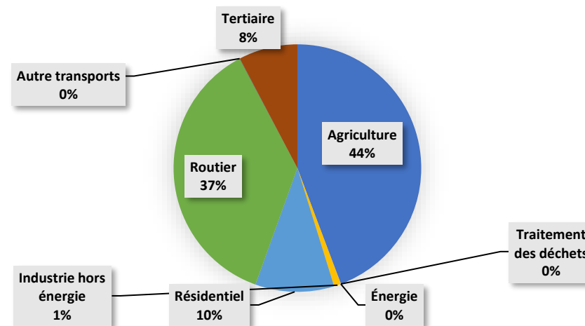
Figure 86 : Répartition des émissions de GES par secteurs en 2021 – Source : Citepa 2021, Inventaire territorialisé des émissions de GES
