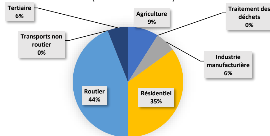
Part de la consommation énergétique en kWh par secteur en 2020 (CC Plaine Jurassienne)
